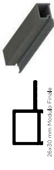
26x30 mm Modulo Partenza
